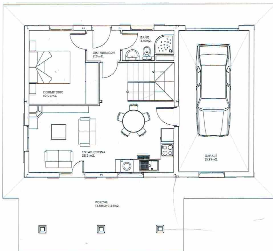
PLANTA BAJA
