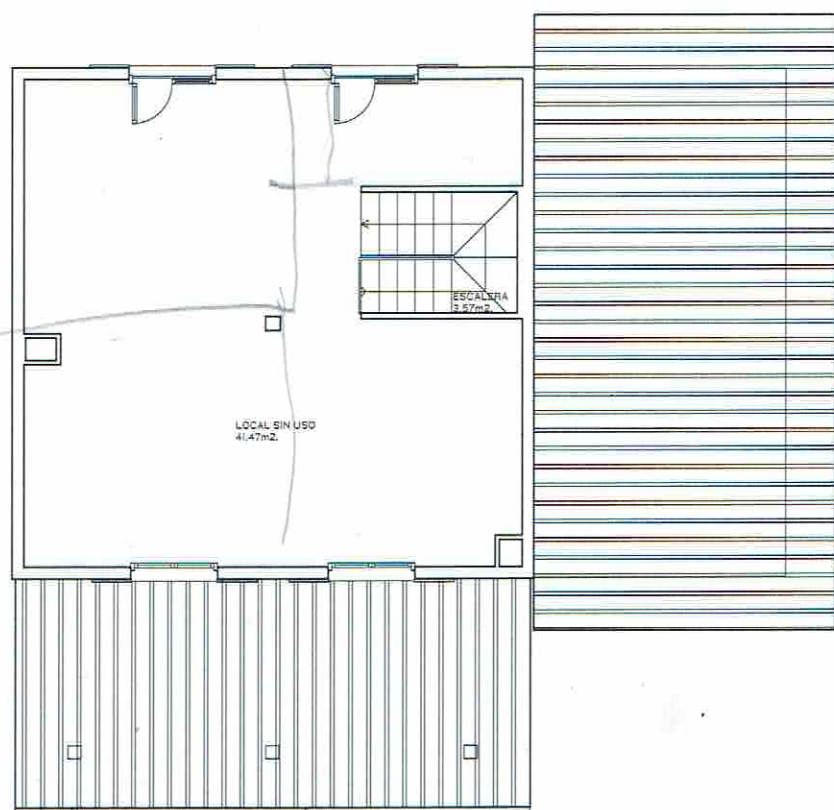
PLANTA PRIMERA
