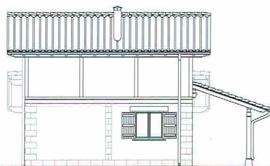
ALZADO NOROESTE
